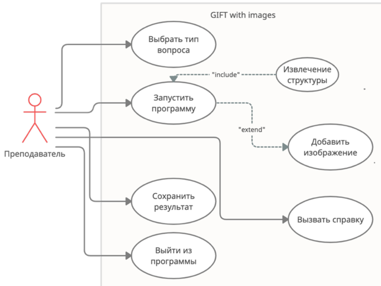
Диаграмма прецедентов разработанного приложения для авторизации создания тестовых заданий.
