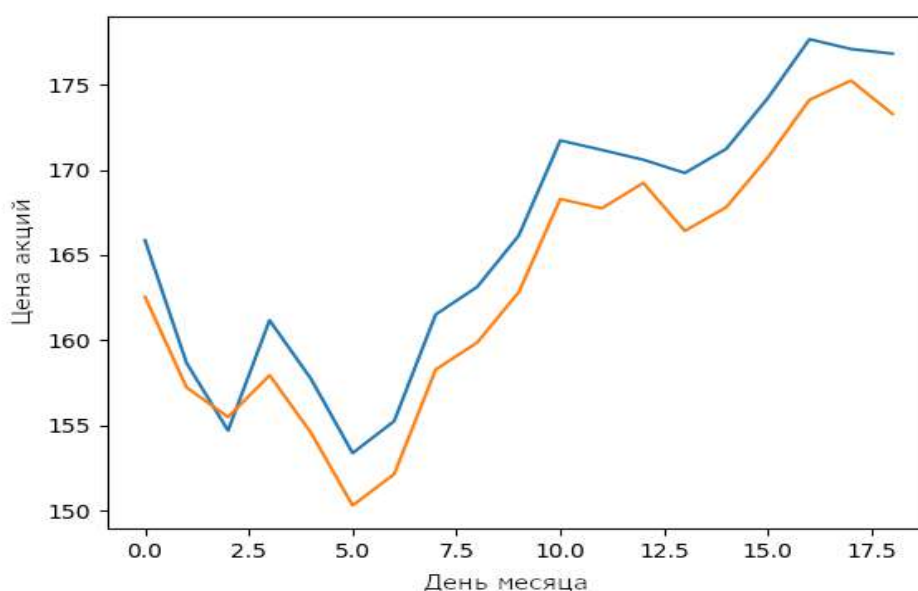
Рисунок 3. Прогноз модели LSTM на цены акций Apple в феврале.
