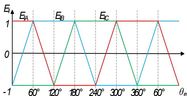
Рисунок 1. Форма сигналов противо-ЭДС электрического угла поворота ВД.
