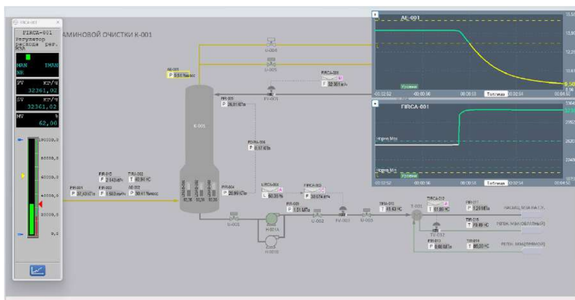
Рисунок 3. Влияние увеличения расхода МЭА на содержание сероводорода в отходящем газе.
