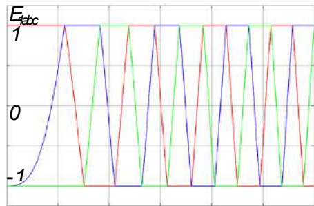
Рисунок 7. Формирование единичных сигналов противо-ЭДС.
