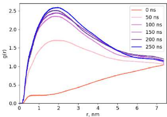
Рисунок 4. RDF Dps-антибиотик, 55°C.
