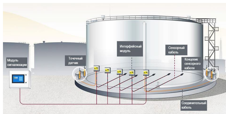
Рисунок 1. Сенсорные системы раннего обнаружения протечек нефтепродуктов.
